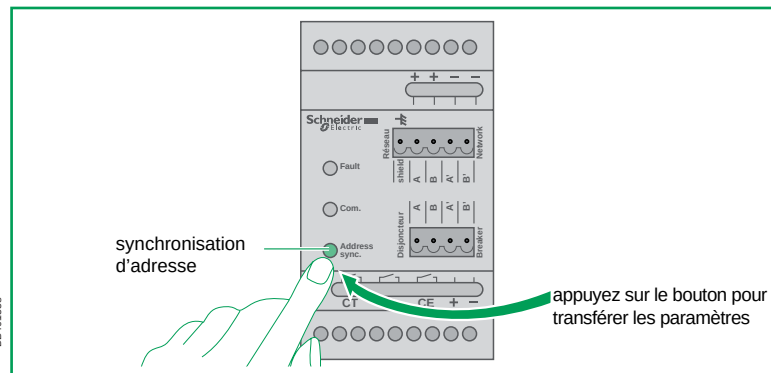
Configuration du module de communication "châssis" CCM Modbus.
