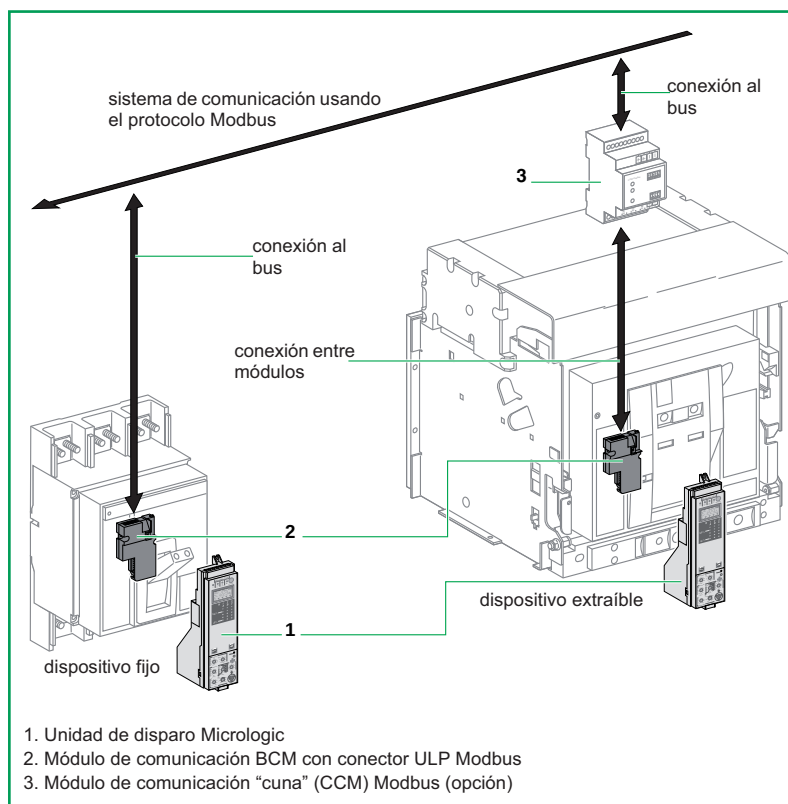
Descripción general de la opción COM.
