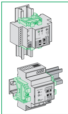
Montage sur rails DIN.
