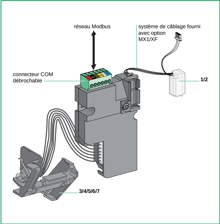
Module de communication "appareil" BCM ULP Modbus et connexions.
