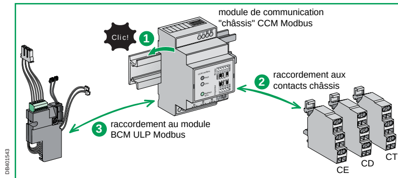
Etapes de l'installation du module de communication "châssis" Modbus sur Compact NS et Masterpact NT/NW débrochables.
