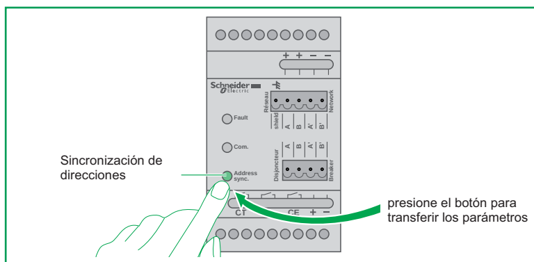
Configuración del módulo de comunicación “cuna” (CCM) Modbus.
