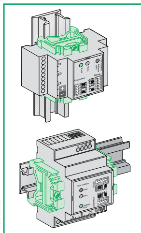
Montaje en riel DIN
