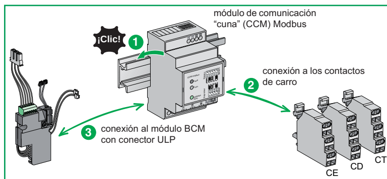
Pasos para instalar el módulo de comunicación “cuna” (CCM) Modbus en los Compact NS extraíbles y Masterpact NT/NW extraíbles
