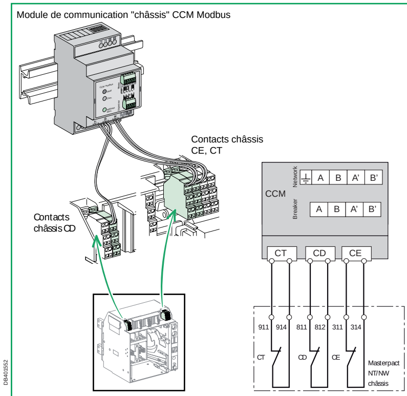
Connexion aux contacts châssis.
