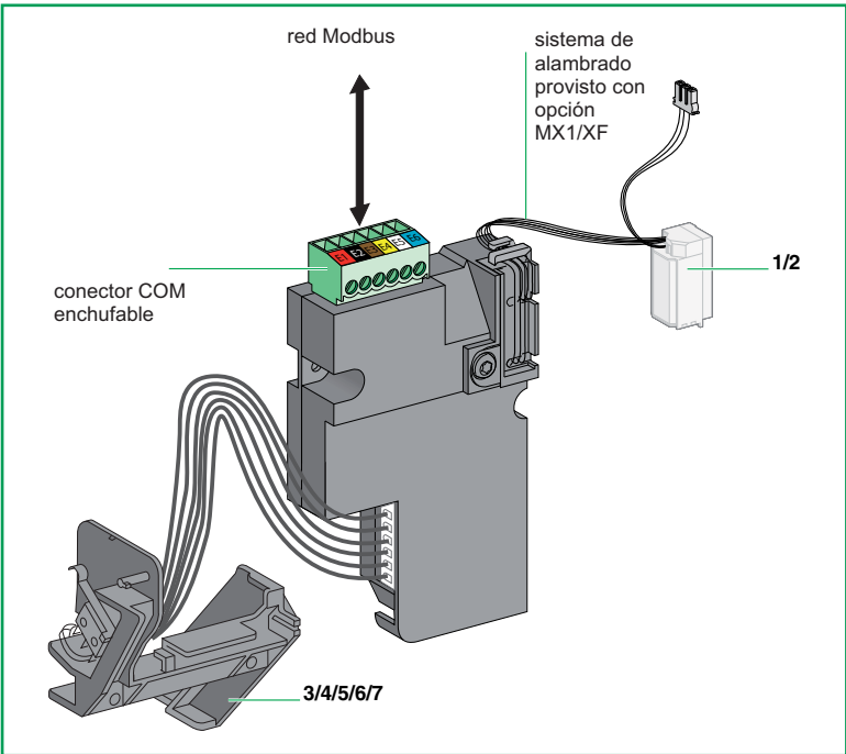
Módulo de comunicación BCM con conector ULP Modbus y conexiones
