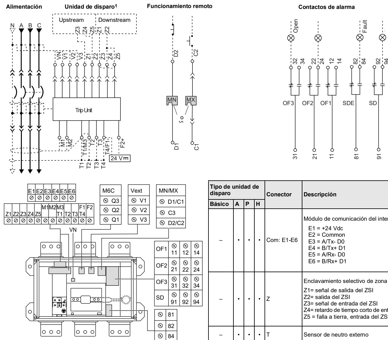
FIG. 3 : Diagramas del cableado de control de los accesorios (Espanol)
