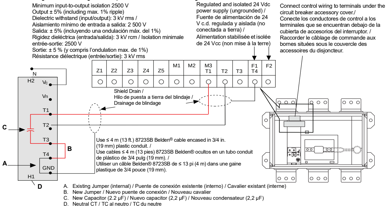
FIG. 6 : Wiring Schematic / Diagramas esquemáticos / Schéma de câblage
