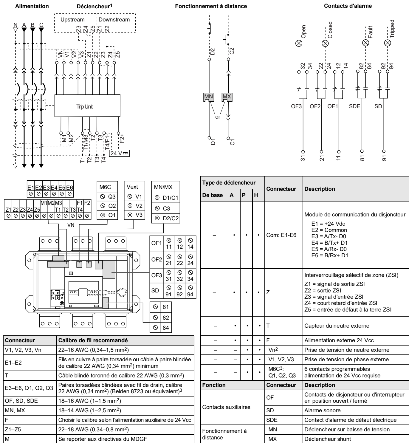
FIG. 4 : Schémas de câblage de commande des accessoires pour disjoncteurs à commande manuelle (Français)
